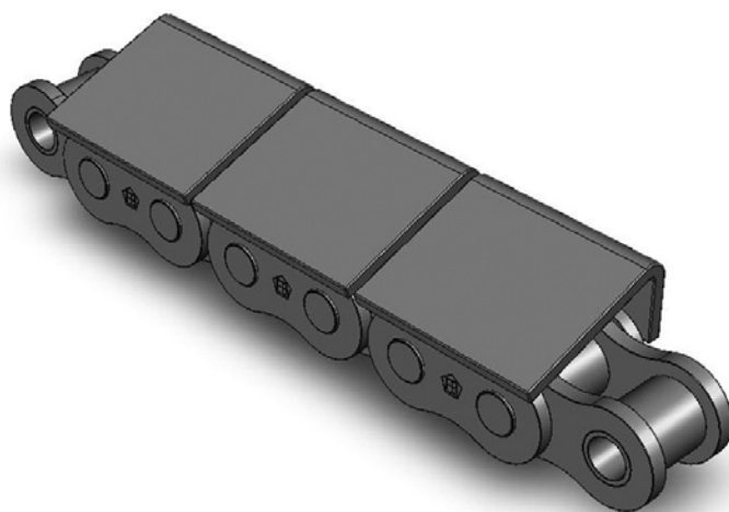
Sågverkskedja med snedtak, 24B-1
