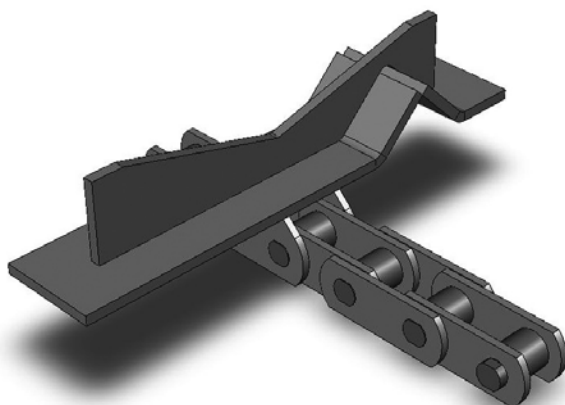
Kerattkedja med medbringarstyrning
